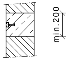
Detail Ankerschiene M 1:20
