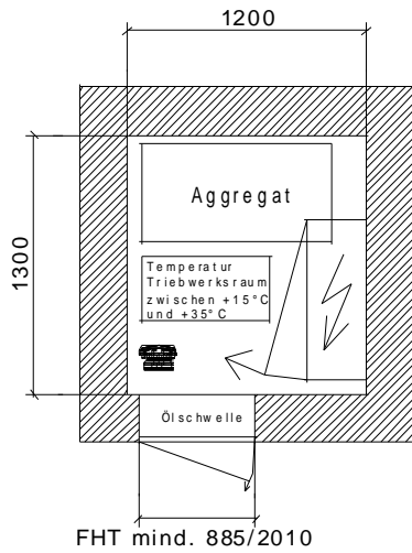
Triebwerkraum (z. B. unter dem Treppenlauf) TWR min. 2000 hoch
