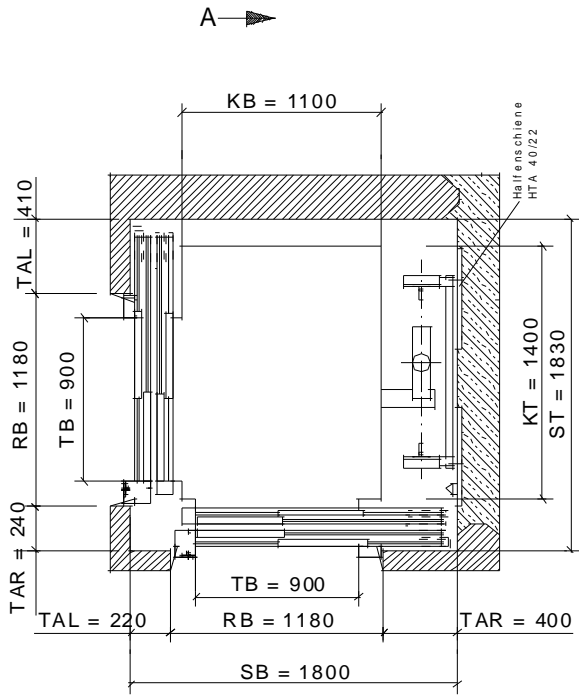
Schachtgrundriss
