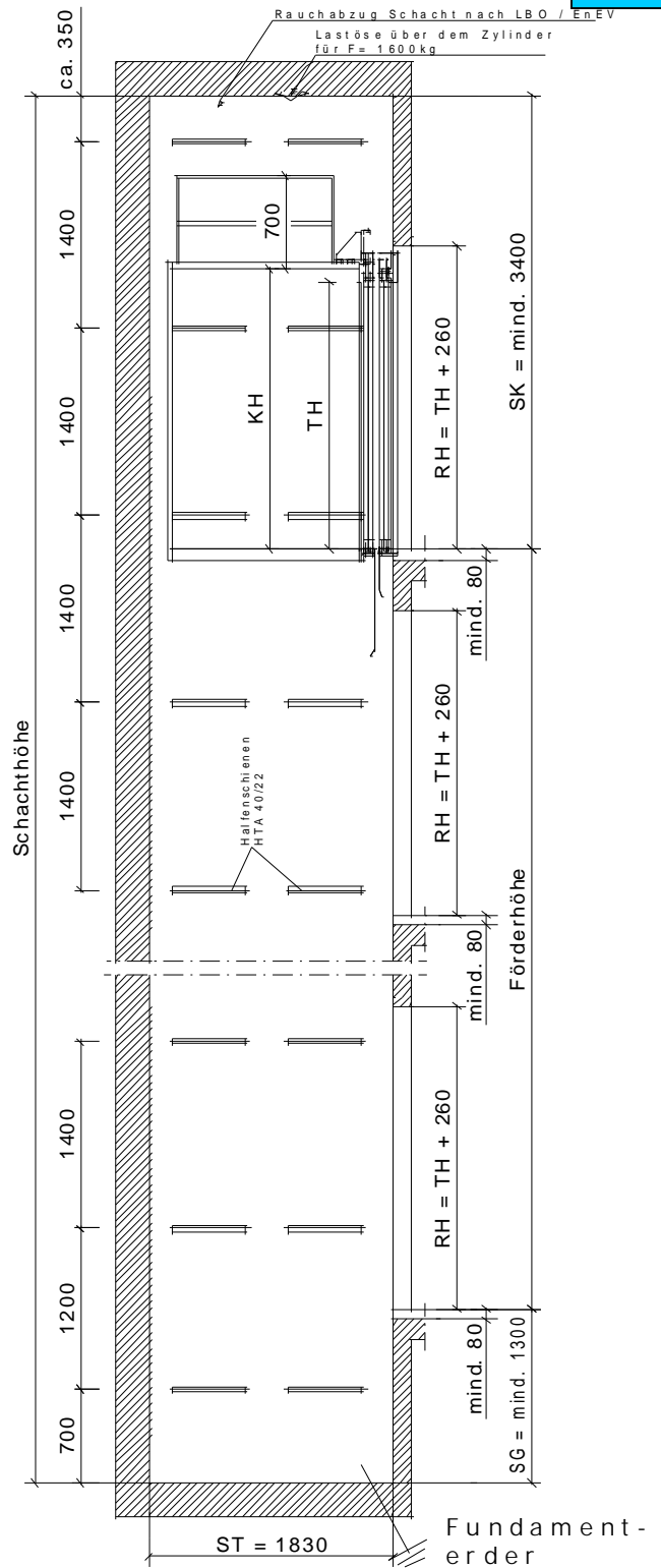
Schnitt A-A
