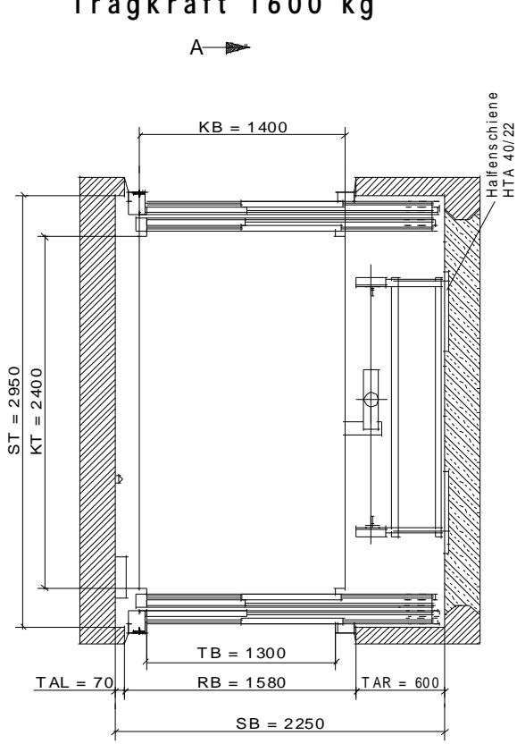
Schnitt A-A Schachtgrundriss
