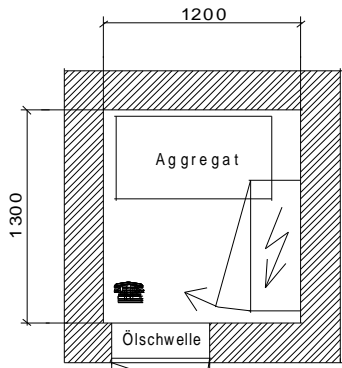
Schnitt A-A Schachtgrundriss
