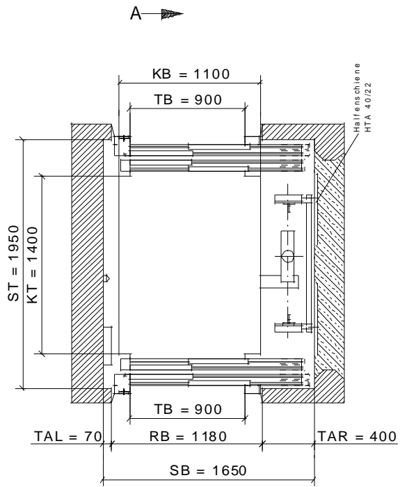
A → Schachtgrundriss
