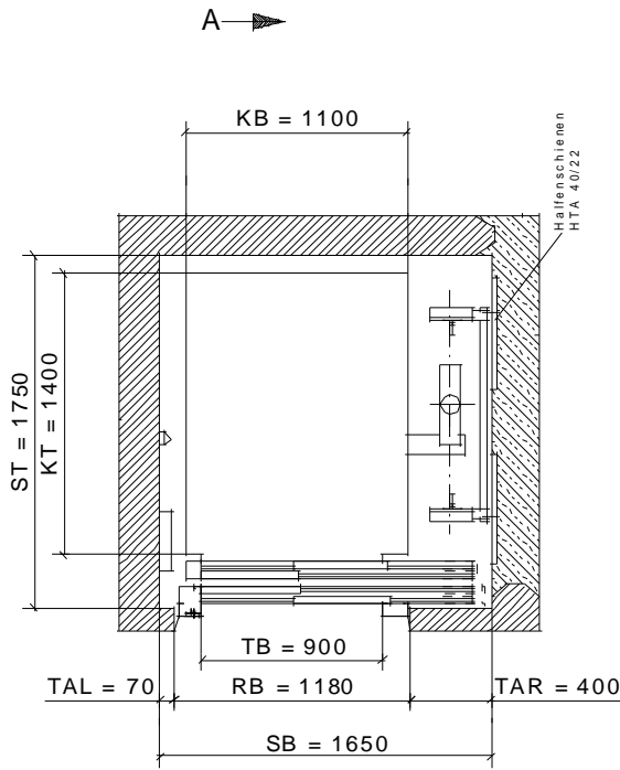
Schachtgrundriss
