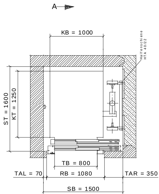
Schachtgrundriss
