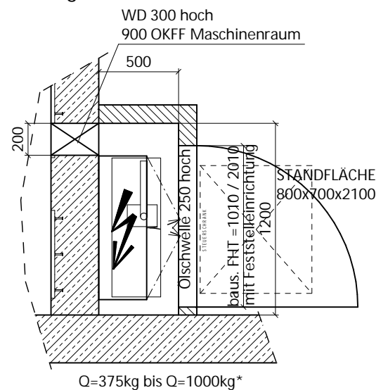
Schachtgrundriss
