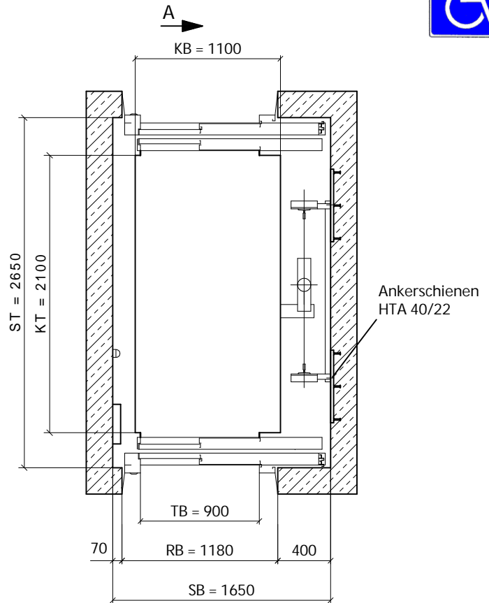
Schachtgrundriss
